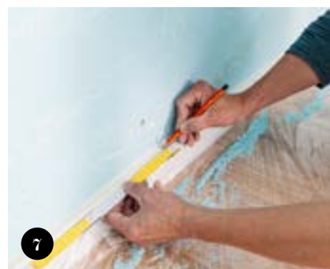
7 Για τα τμήματα διαφορετικού χρώματος σημαδέψτε τα σημεία αρχής και τέλους των διαχωριστικών γραμμών.
