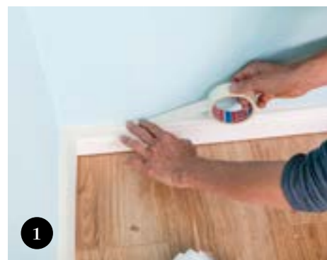
1 Καλύψτε πρώτα με ταινία την επάνω ακμή των σοβατεπί. Αφήστε την ταινία να προεξέχει λίγο προς τα κάτω.
