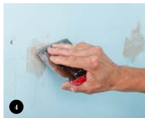
4 Στοκάρετε τώρα όλες τις τρύπες. Βρέξτε ελαφρά τις μεγαλύτερες τρύπες για να «πιάσει» καλύτερα στον σοβά ο στόκος.
