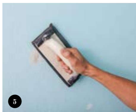
5 Αφήστε να στεγνώσει παντού ο στόκος και μετά τρίψτε τον τοίχο, προσέχοντας να ασκείτε παντού ίδια περίπου πίεση.
